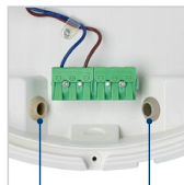
Einfache Weiterverdrahtung
