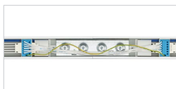
Sehr stabile Kupplung zwischen den Tragschienen für lange Abhängeabstände von bis zu 4,6 m
