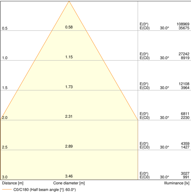
HB DA P 150W 840 70DEG IP66
