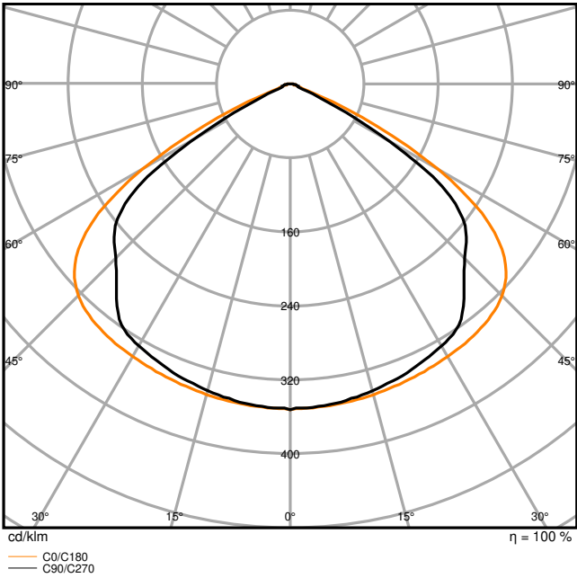
LB FLEX 1500 P 140W 840 VW
