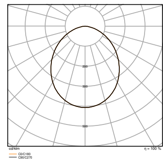
DL CMFT ZB D200 P 30W 930 OP WT
